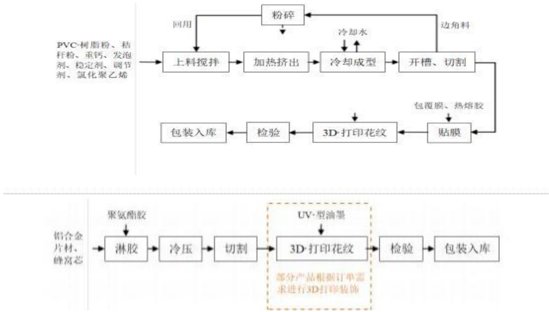
图 2 墙面装饰材料产品生产流程图
